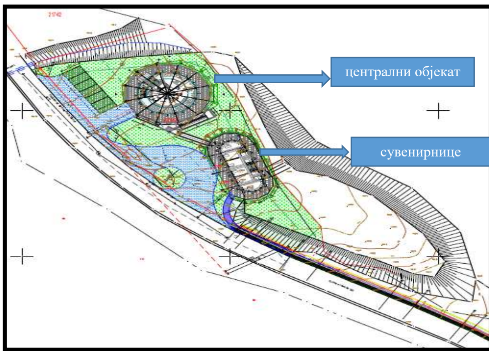
Ситуација основе приземља оба објекта
