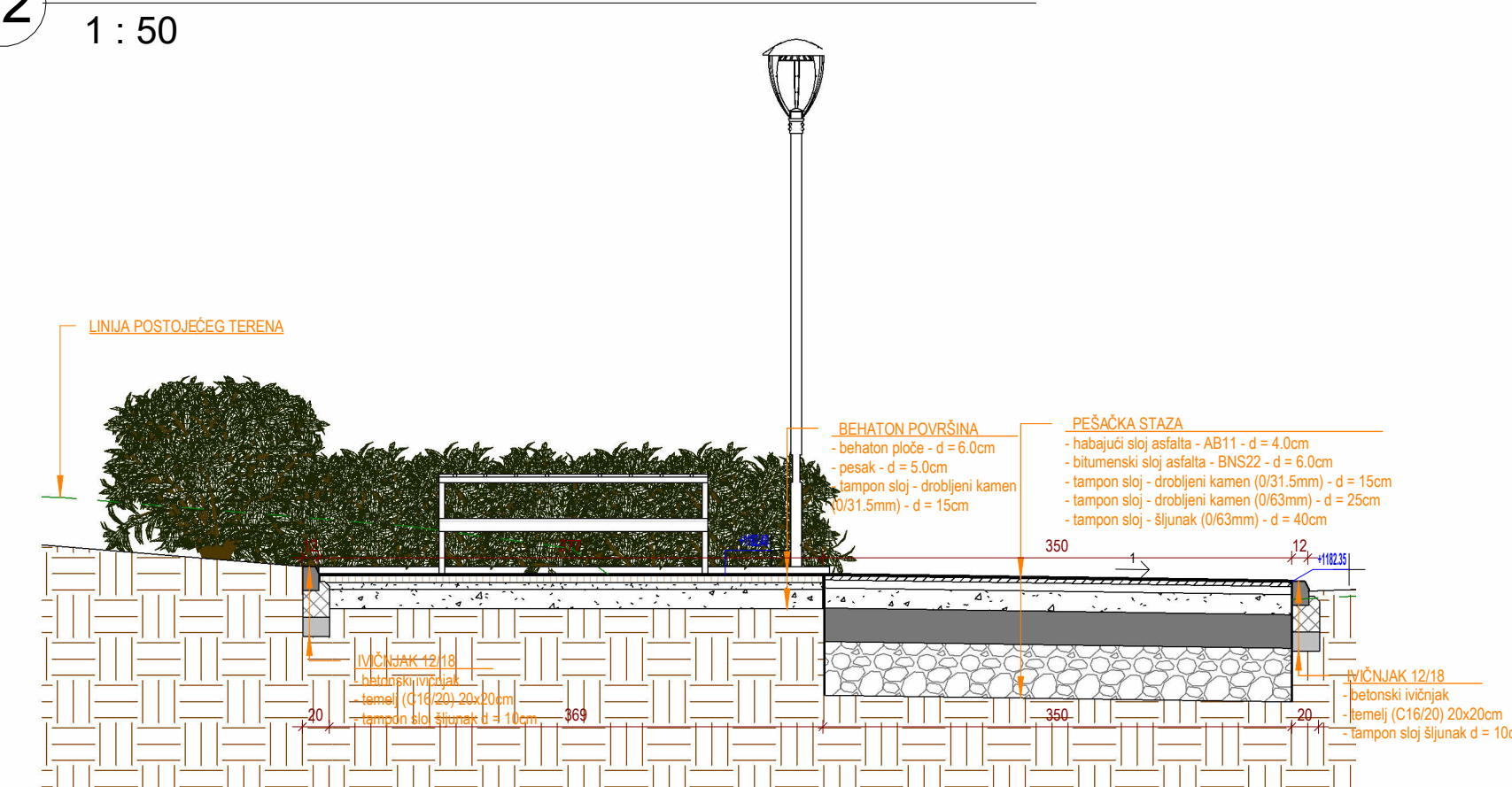
16 Odmorište 6 - presek 1 : 50
