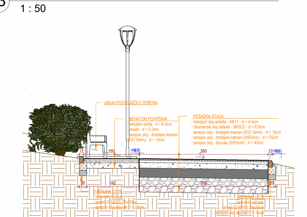
17 Odmorište 7 - presek 1 : 50
