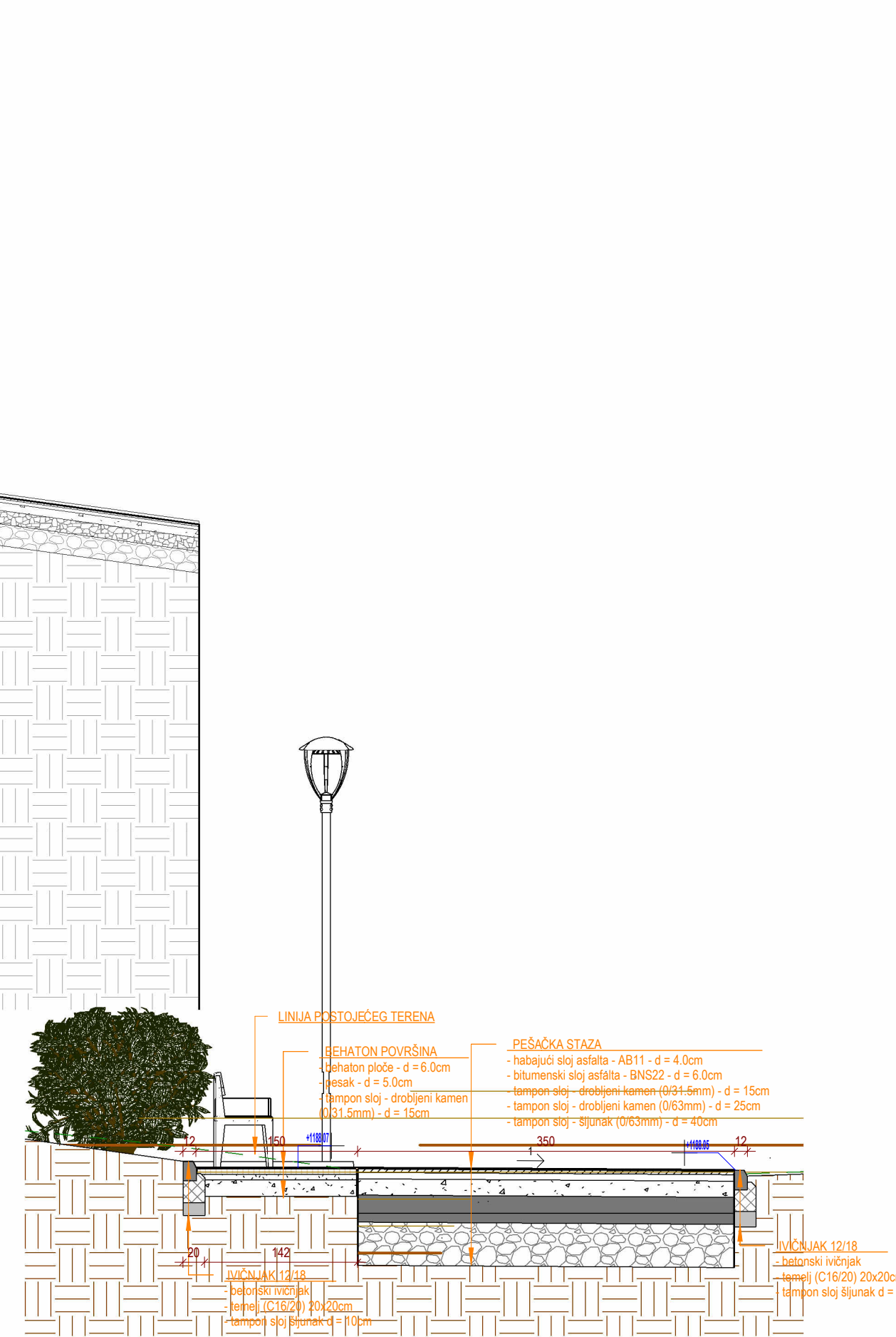
13 Odmorište 3 - presek 1 : 50
