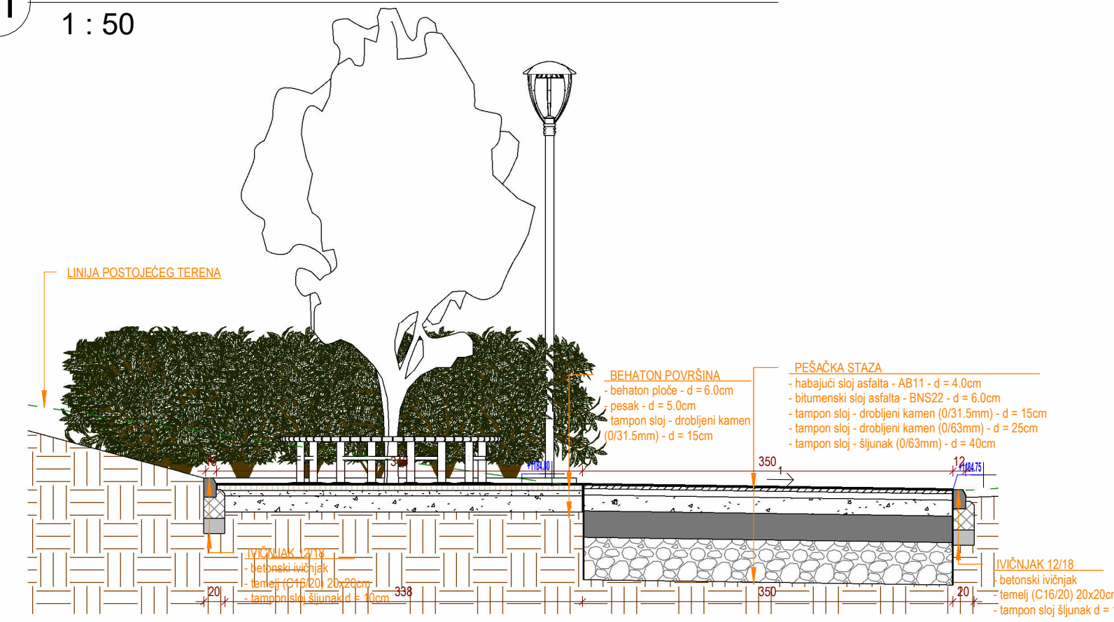
15 Odmorište 5 - presek 1 : 50
