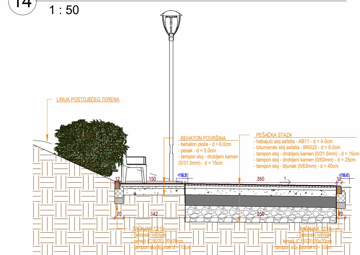
18 Odmorište 8 - presek 1 : 50
