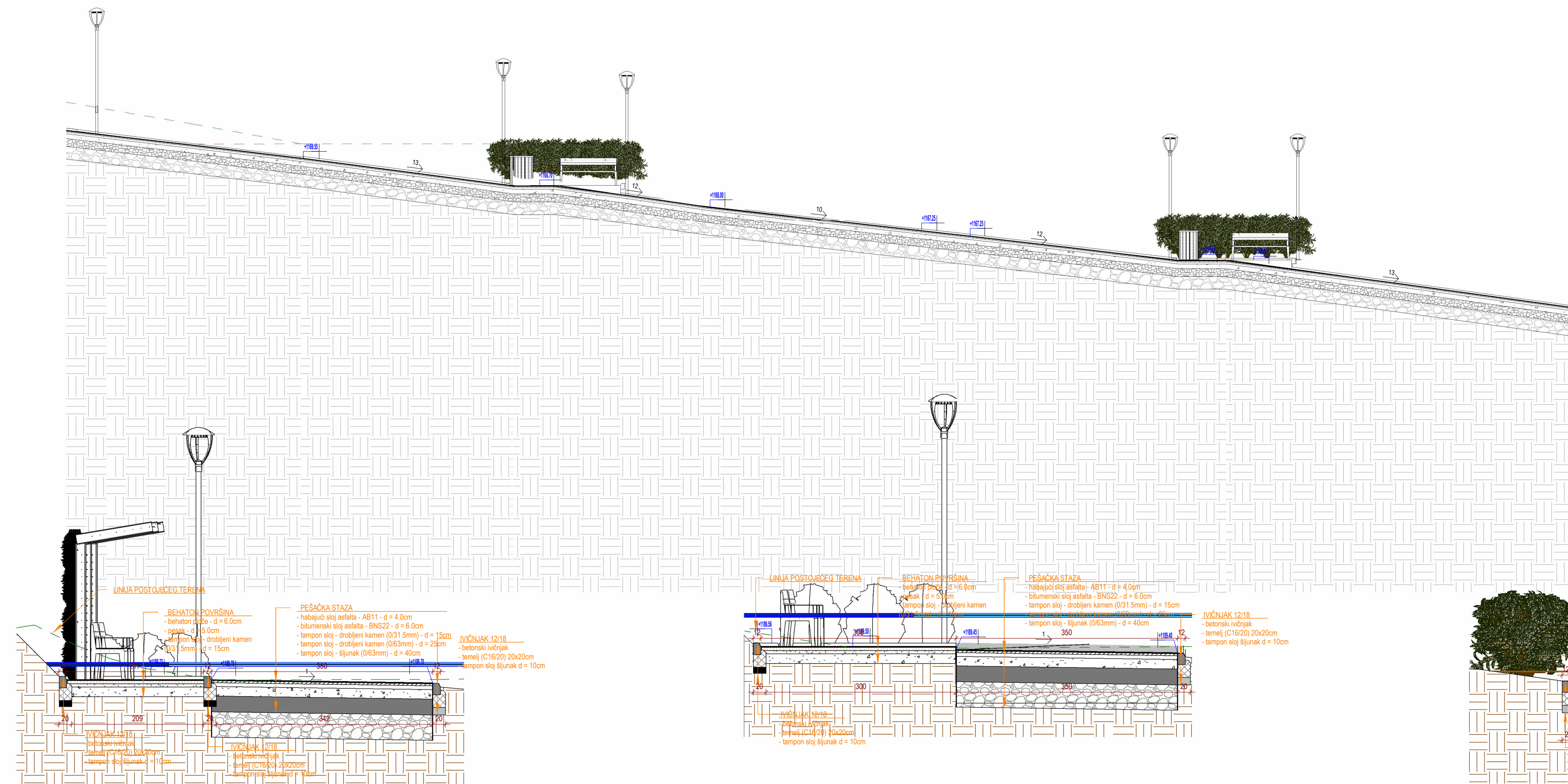
11 Odmorište 1 - presek 1 : 50
